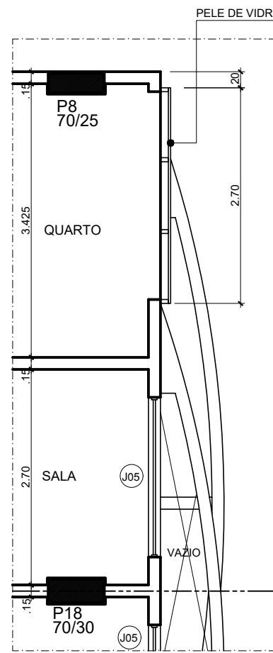
PLANTA BAIXA - PAVTO. TIPO DO 5º ao 8º ESCALA _____
