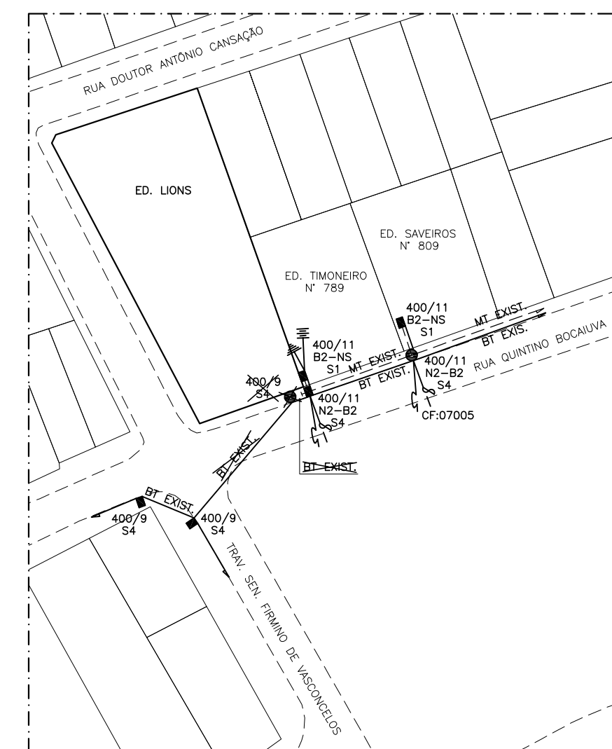
SITUAÇÃO ATUAL - EDIFÍCIO LIONS ESC.: 1/1000
