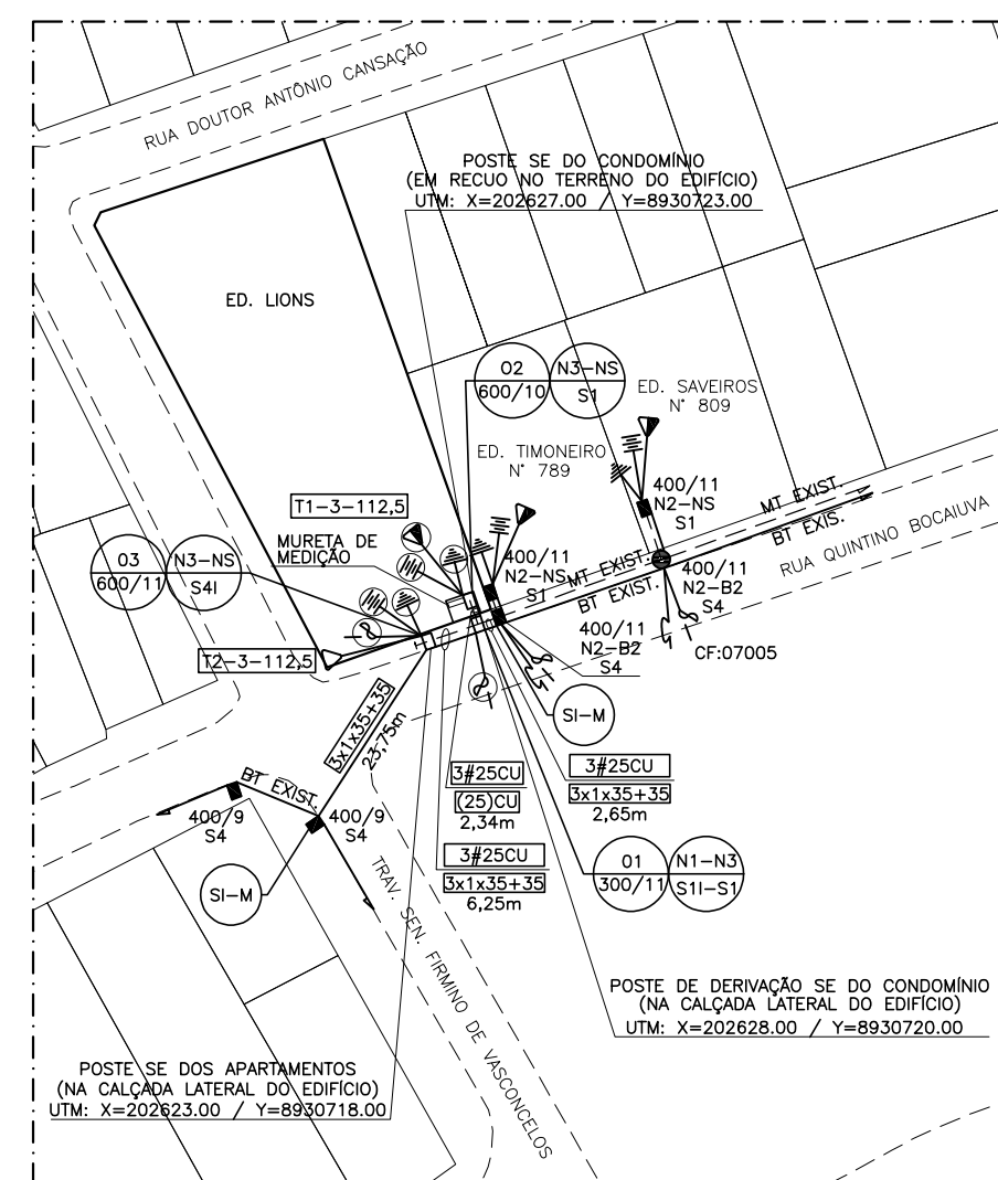
SITUAÇÃO PROJETADA - EDIFÍCIO LIONS ESC.: 1/1000
