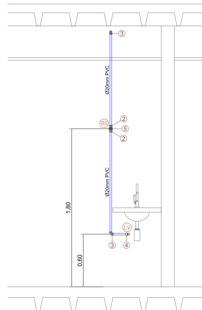
DEE - H.29 ESQ. VERT. RAMAL ALIMENTAÇÃO ESCALA = 1 : 25
