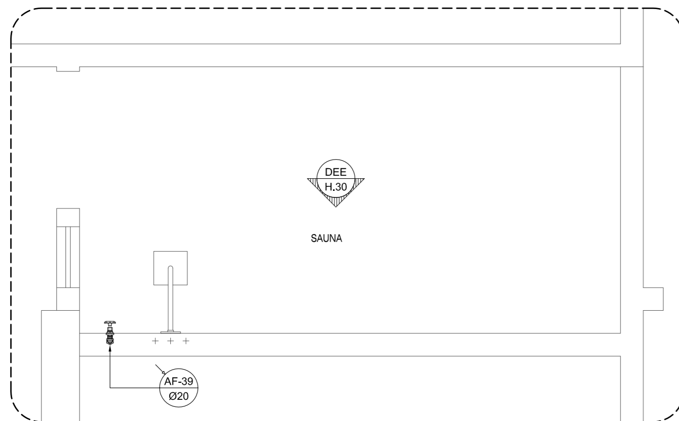
PLANTA BAIXA PILOTIS LAZER - SAUNA ESCALA = 1 : 25
