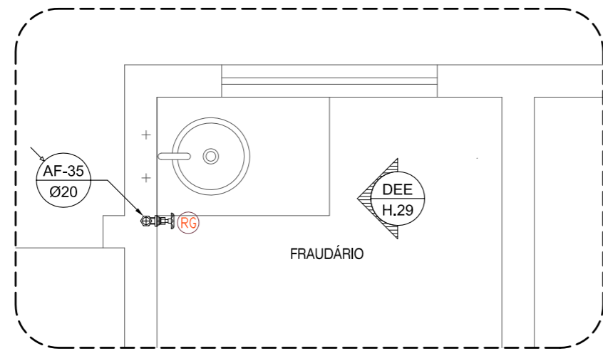
PLANTA BAIXA PILOTIS LAZER - FRAUDÁRIO ESCALA = 1 : 25
