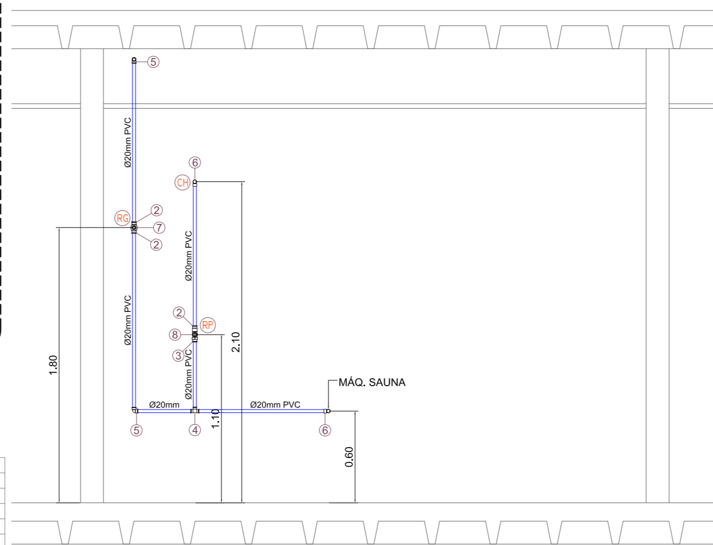
DEE - H.30 ESQ. VERT. RAMAL ALIMENTAÇÃO ESCALA = 1 : 25
