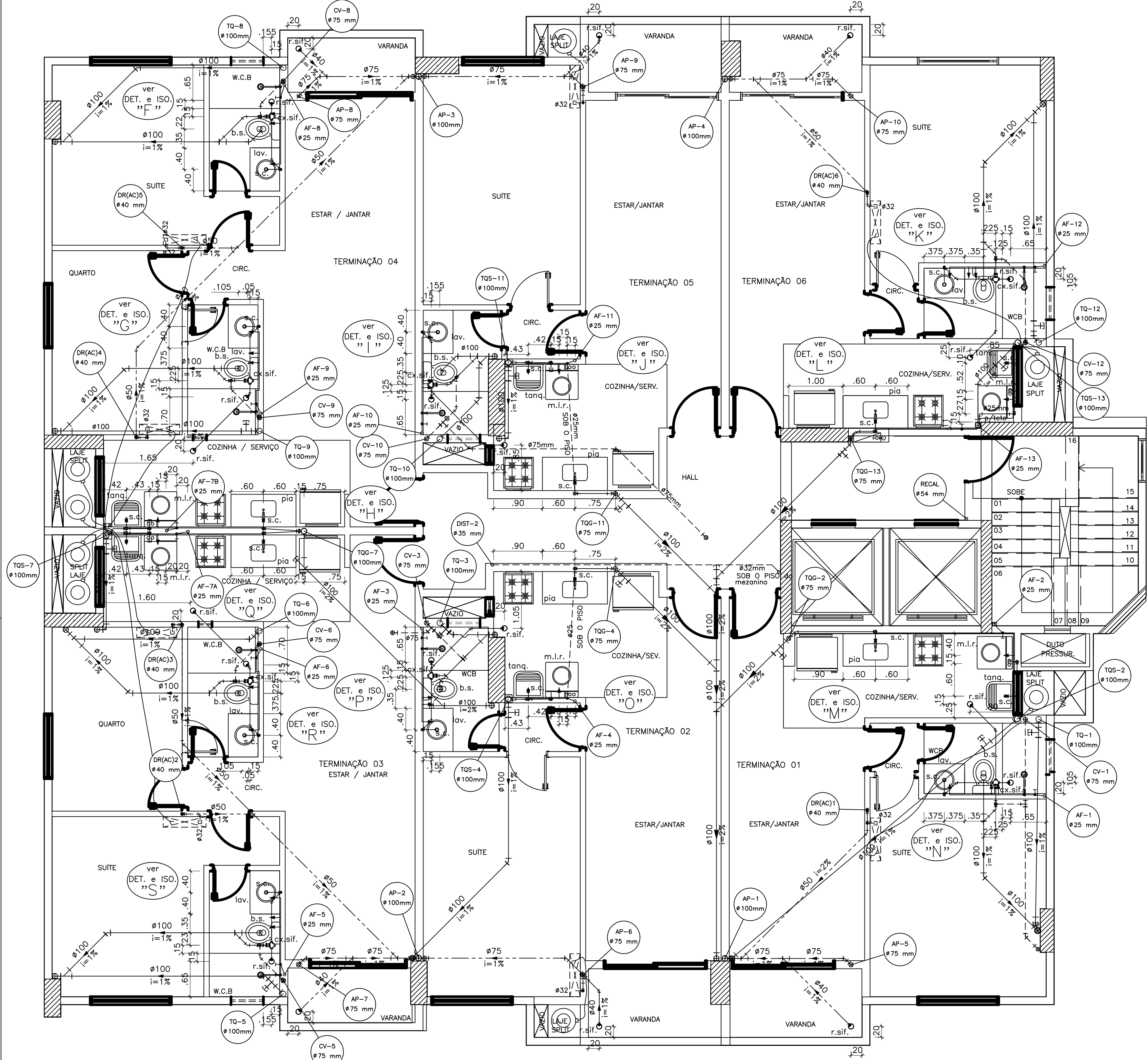
ESQUEMA GERAL - 1º PAVIMENTO ESCALA: 1/50
