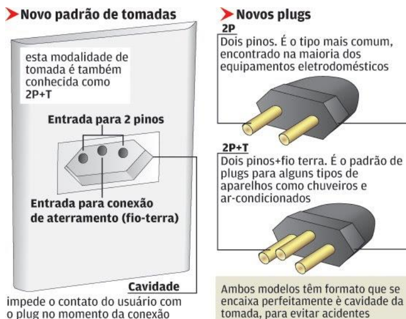
Figura 6 - Novo padrão de tomadas
