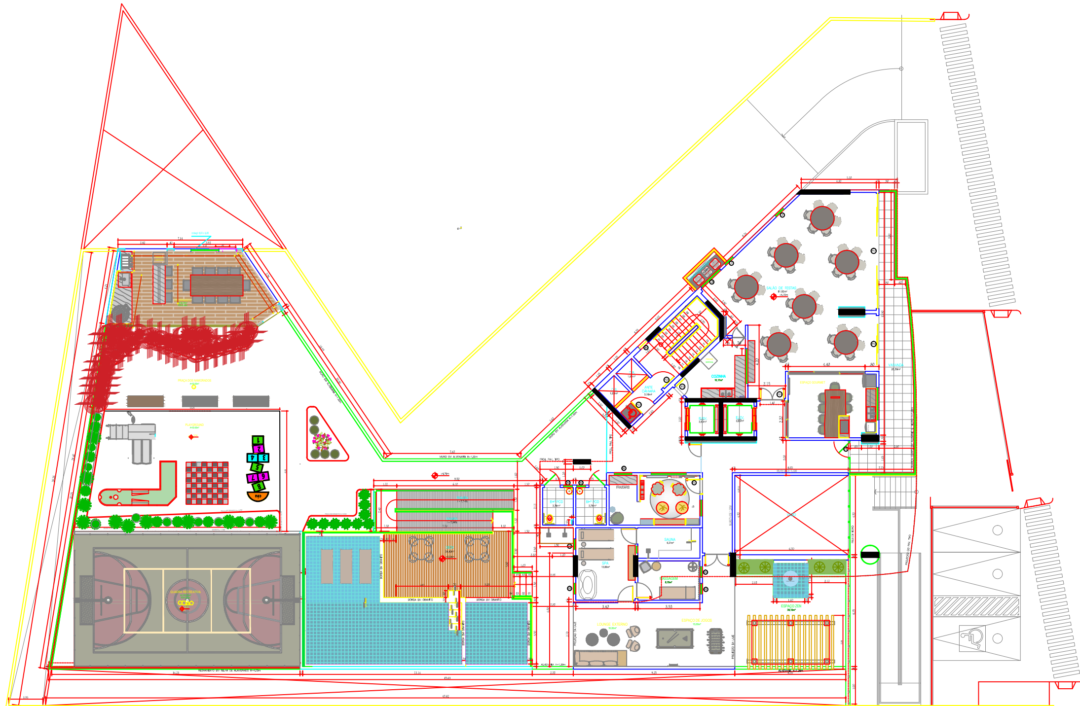
PLANTA BAIXA - PILOTIS LAZER Escala: 1/75
