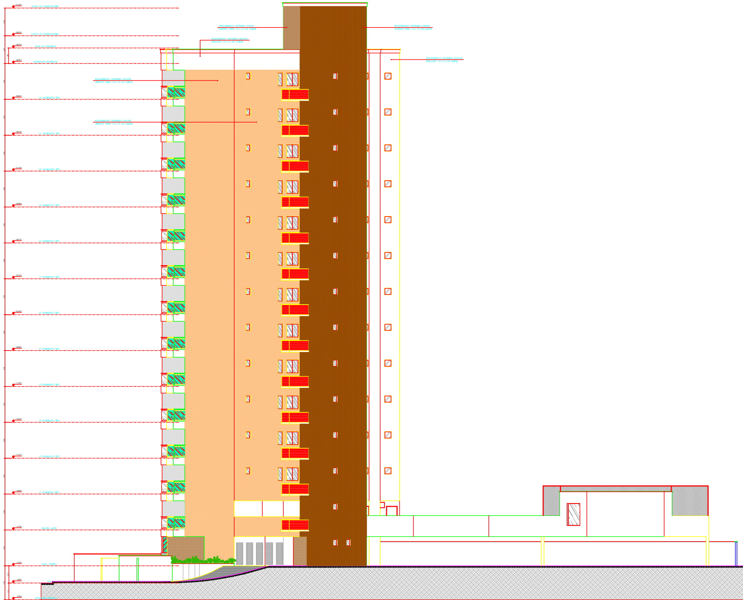
FACHADA LATERAL ESQUERDA Barr. 1/75
